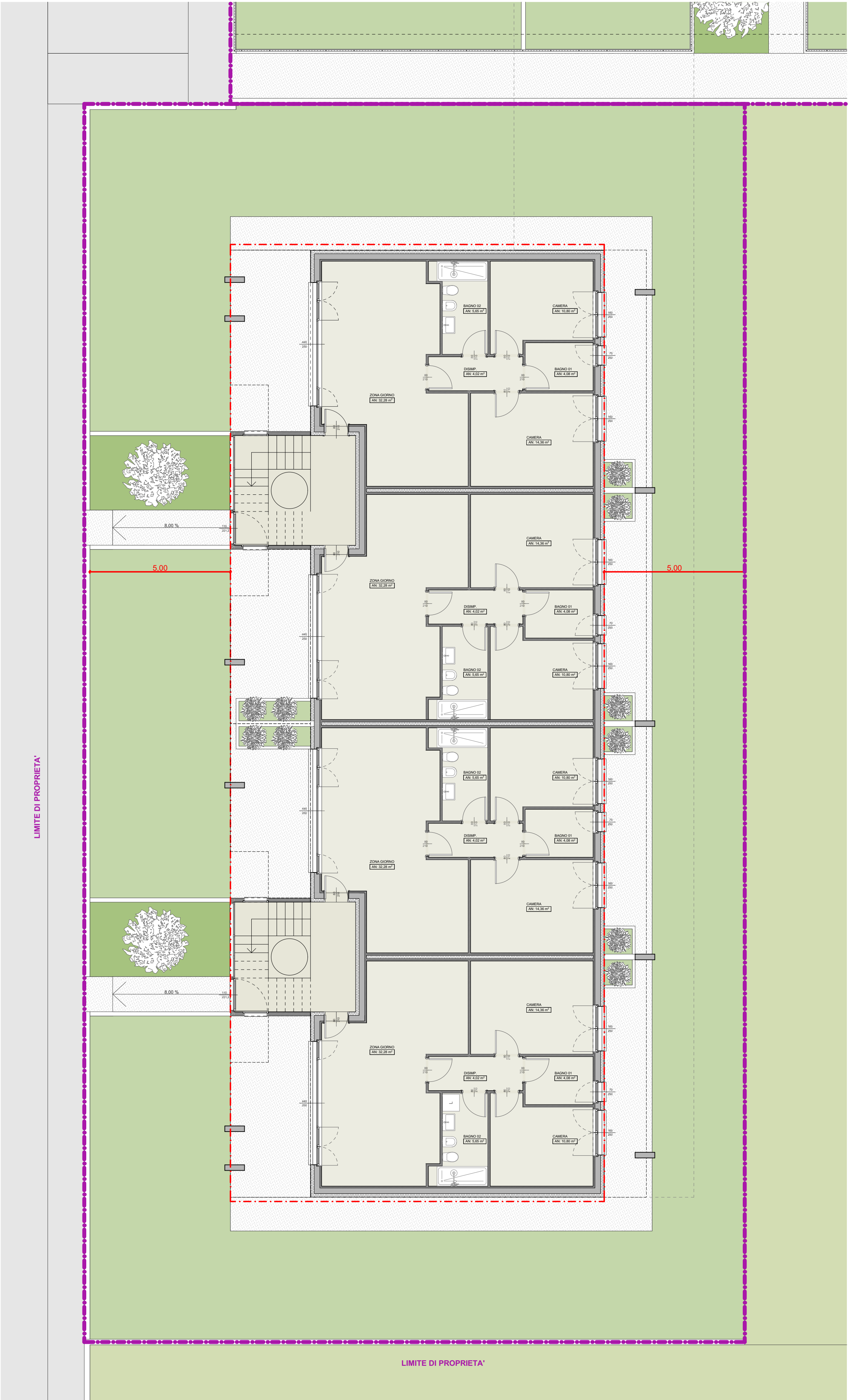
PIANTA PIANO TERRA - BLOCCO A
